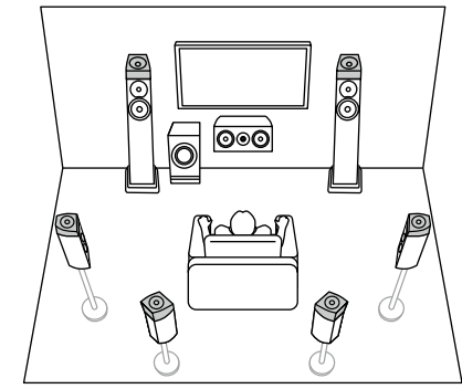
7.1.2 canales (Altavoces con tecnología Dolby (Delanteros o Envolventes o Envolventes traseros)) ( →p30)
