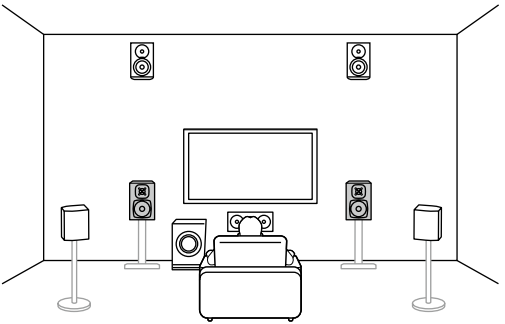
5.1.2 canales (Bi-amplificación (Delanteros)) (→p29)
