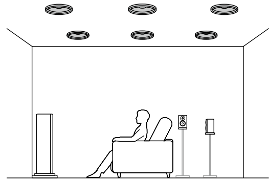
7.1.2 canales (delantero superior o medio superior o trasero superior) ( →p30)
