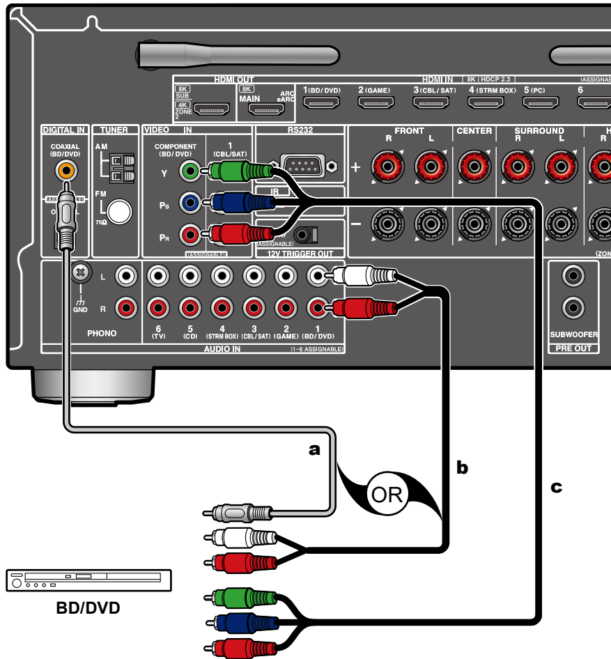
a Cable coaxial digital, b Cable de audio analógico, c Cable de video componente
