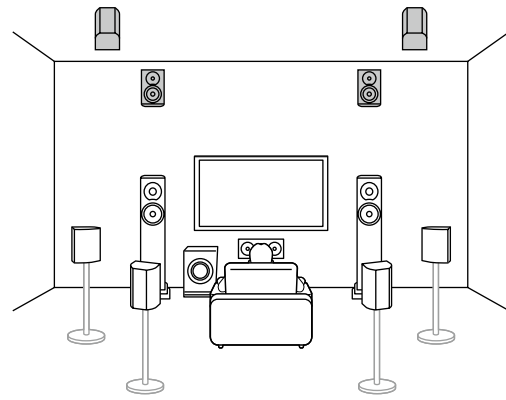
7.1.2 canales (de altura delanteros o de altura traseros) ( →p30)
