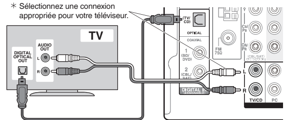
Connexion avec un téléviseur qui n'est pas compatible avec la fonction ARC
