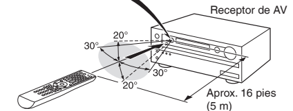
Sensor del mando a distancia
