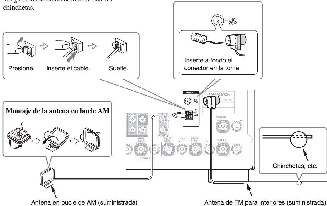
Antena en bucle de AM (suministrada)
