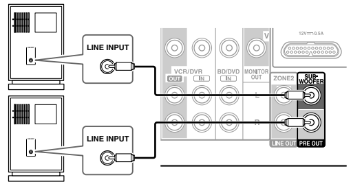
Subwoofer amplifié
