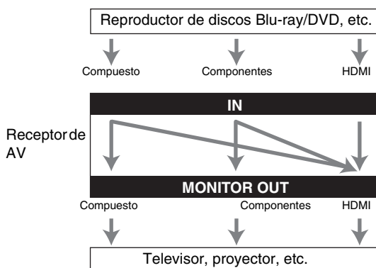
Gráfico de flujo de señal de vídeo
