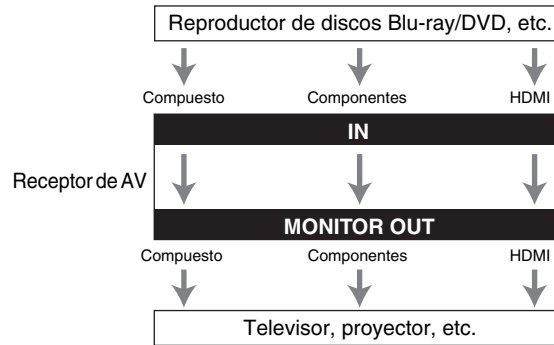
Gráfico de flujo de señal de vídeo
