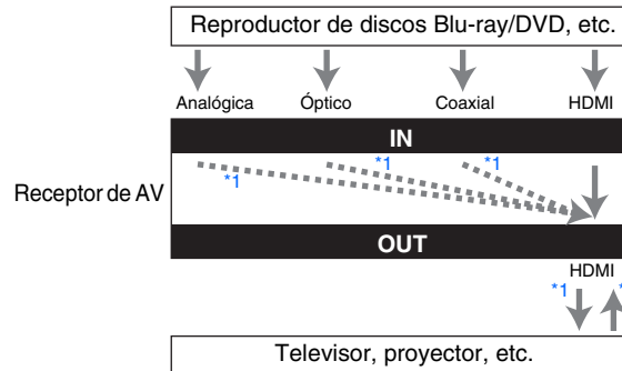
Gráfico de flujo de señal de audio
