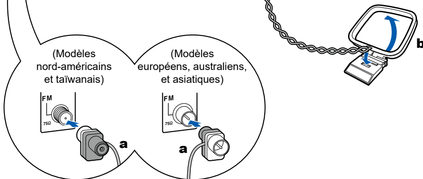
a Antenne FM intérieure, b Antenne cadre AM
