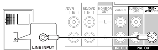
Subwoofer amplifié
