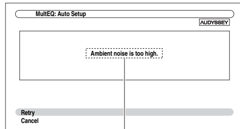
Error message
