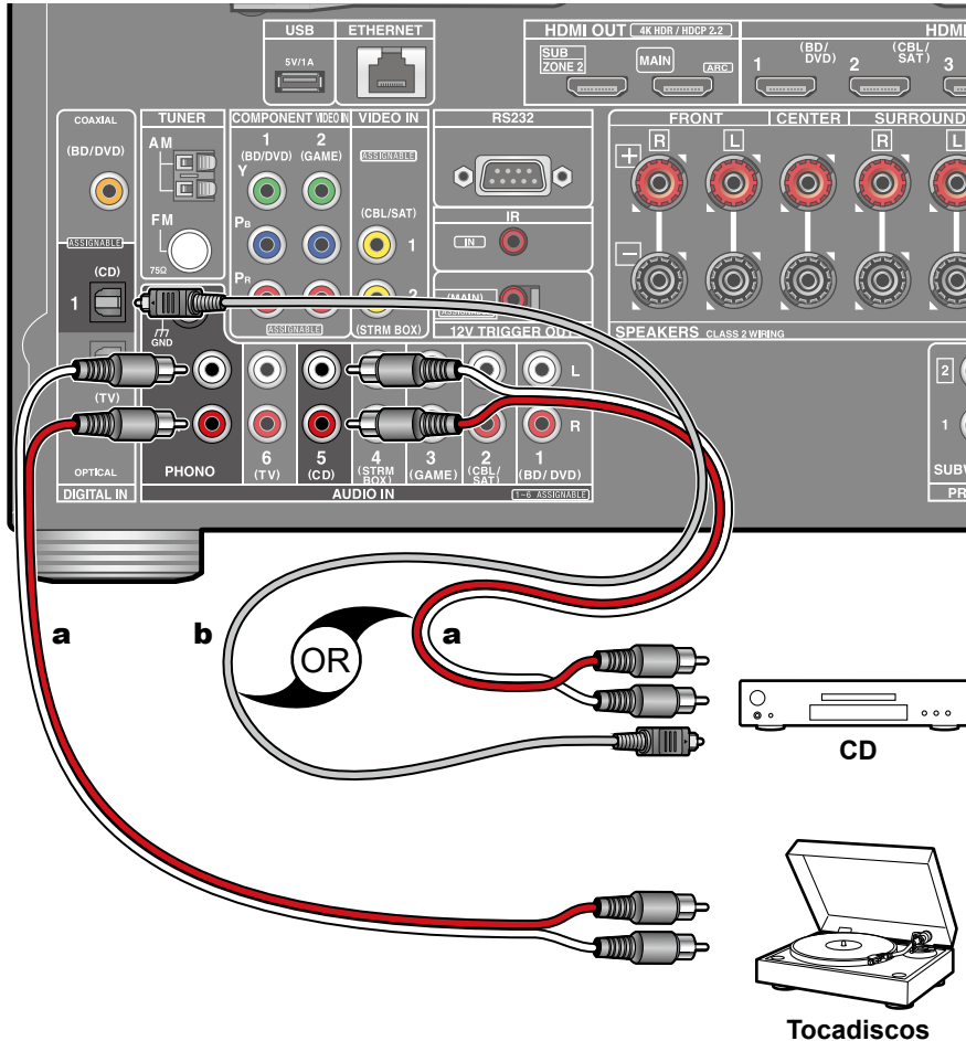
a Cable de audio analógico, b Cable óptico digital
