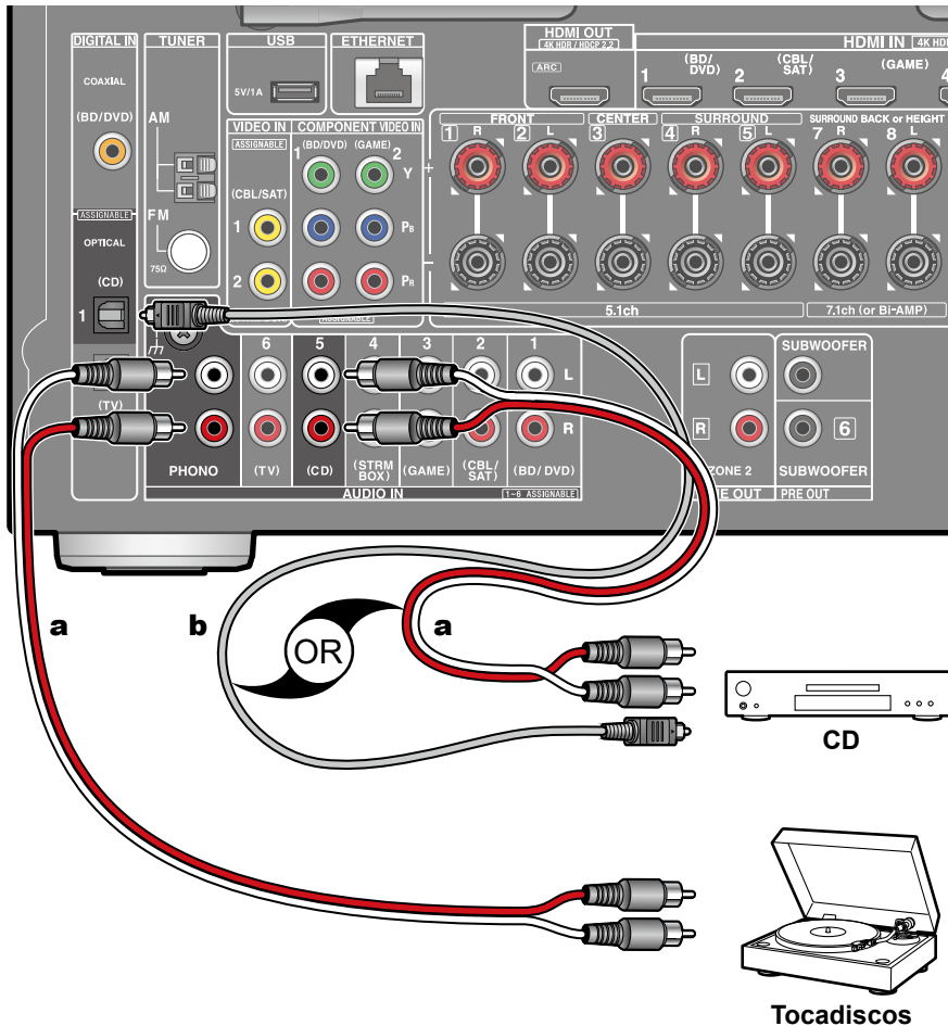
a Cable de audio analógico, b Cable óptico digital
