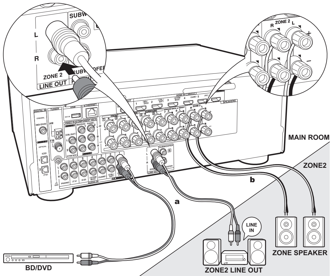
a Cable de audio analógico, b Cable de altavoz
