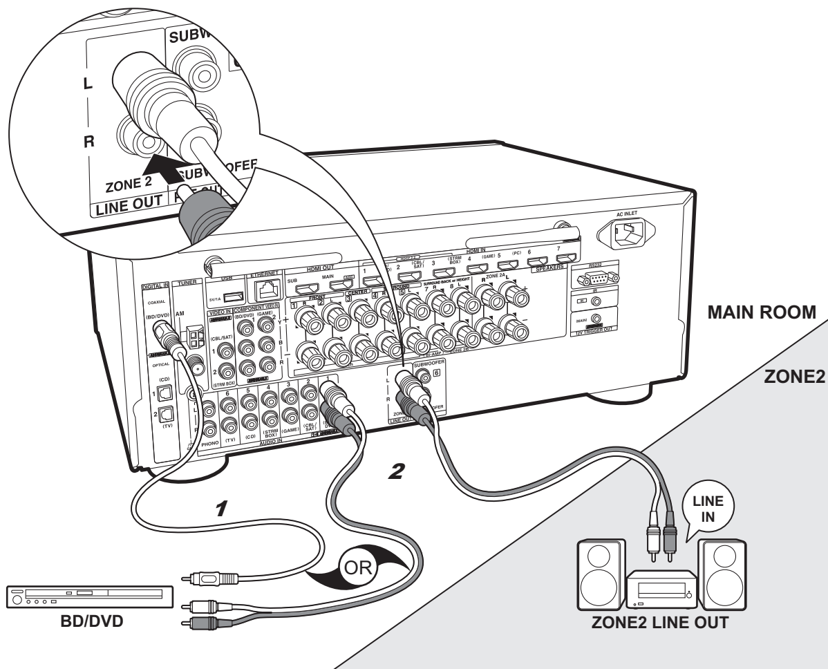
1 Cable coaxial digital, 2 Cable de audio analógico
