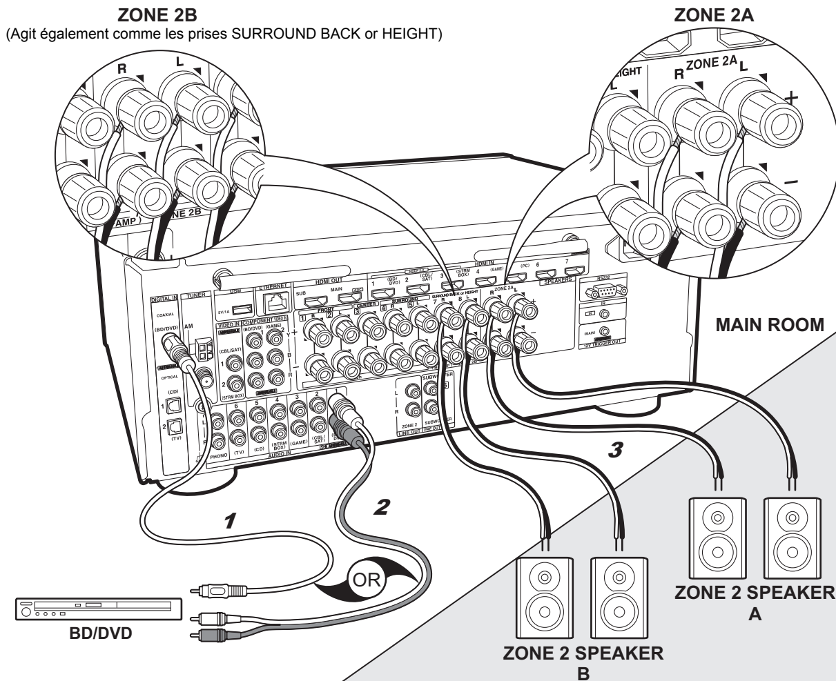
1 Câble coaxial numérique, 2 Câble audio analogique, 3 Câble d'enceinte
